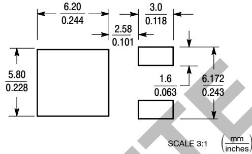
DPAK
